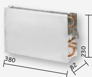
PAROWNIK LAMELOWY VD-03 DO AGREGATÓW SERII 80
